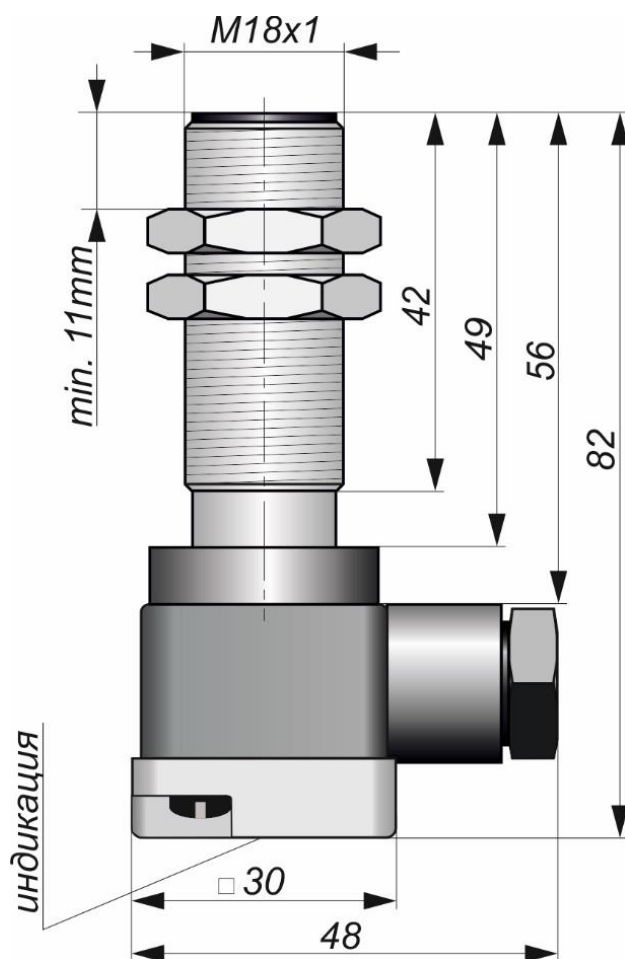
Габаритный чертеж
